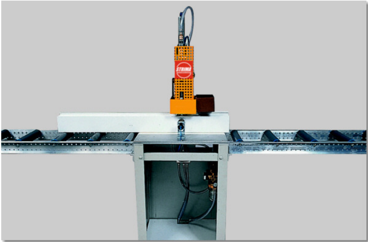
Tischschraubgerät 2954 mit Maschinenfuß und Rollenbahn links und rechts.
